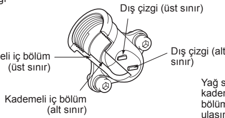
Şekil 2 Yağ borusu
