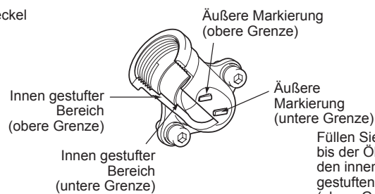
Abb. 2 Ölleitung
