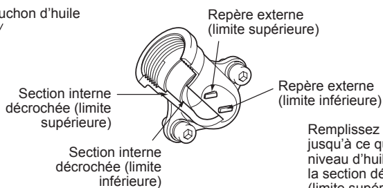
Fig. 2 Tuyau d'huile
