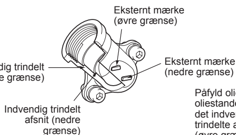
Fig. 2 Olierør
